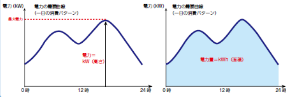
図Ⅱ-2-1 電力と電力量のイメージ（電力需要曲線）
